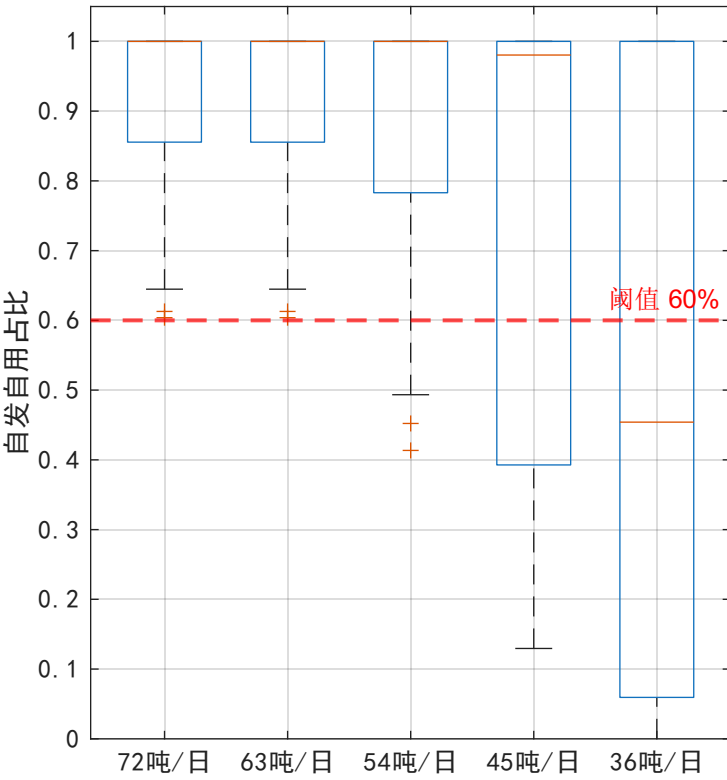
图 6(a) 新能源自发自用电量占比
