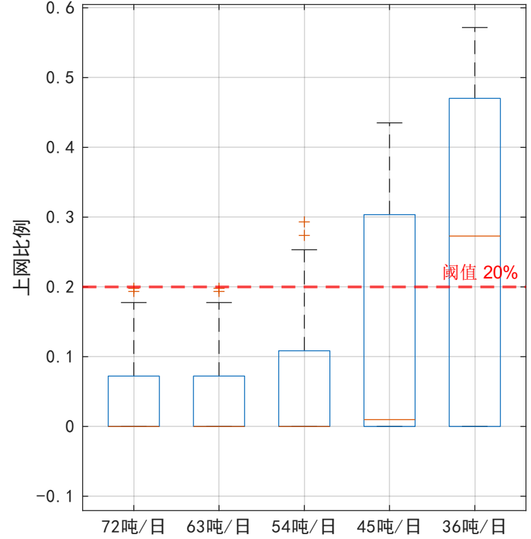
图 6(c) 新能源上网电量比例
